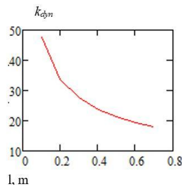
3 pav. Dinamiškumo koeficiento priklausomybė nuo ilgio
