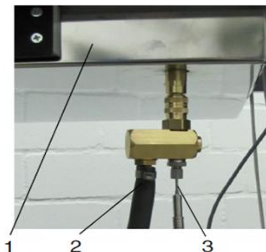
6 pav. Temperatūros matavimas
