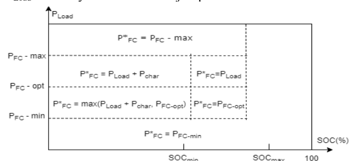
2 pav. Skraidyklių autopilote numatytas optimalus energijos paskirstymo algoritmas – „Rule-based algorithm“
